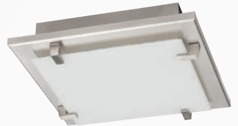
32129/17/10 ↑91 → 320 ↗320 2xE27, max. 23W, 230V, IP20 Včetně zdroje |
